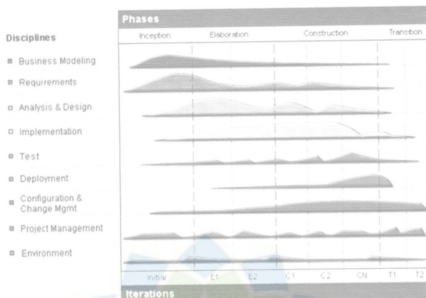
Gambar 1. 2 Metode RUP [16].
