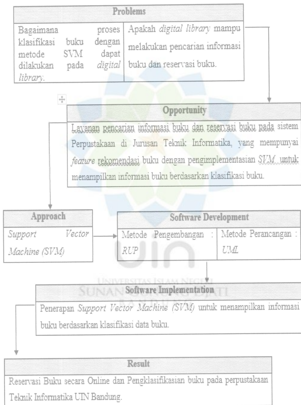
Gambar 1. 1 Kerangka Pemikiran.
