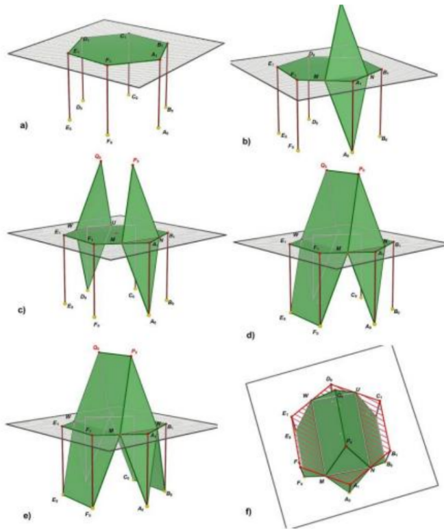
Gambar 2. Urutan Tahapan Konstruksi Alas Tunggal Sarang Lebah (Vallo, Rumanova, Durus, 2014)
