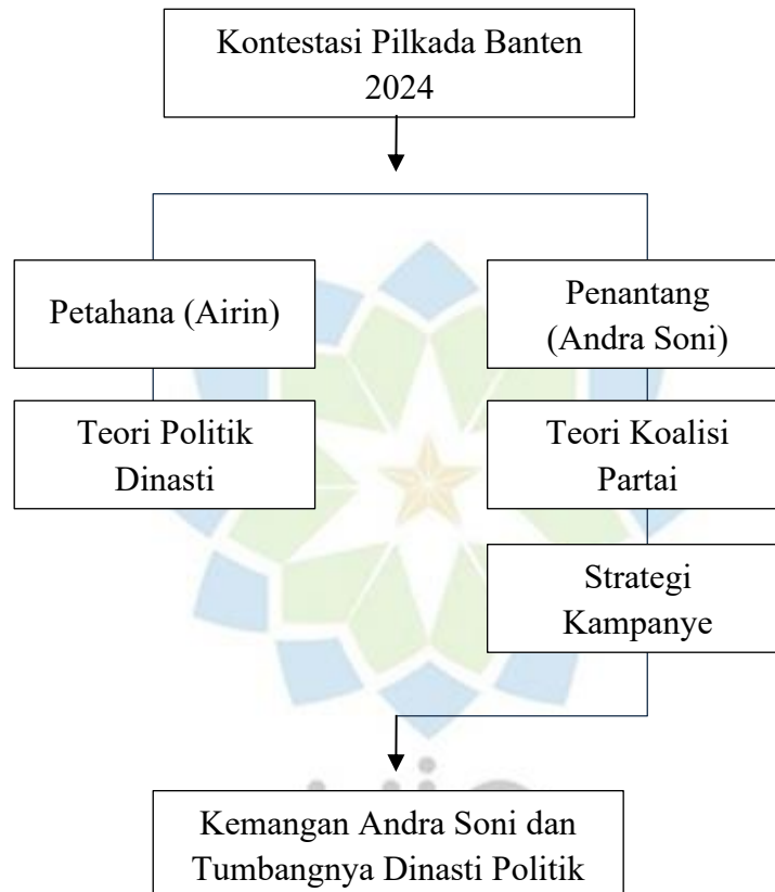
Gambar 1. 1 Kerangka Berpikir
