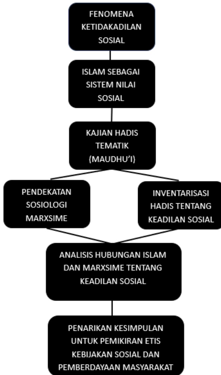
Gambar 1 Kerangka Berpikir
