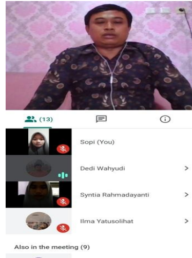
Gambar 1.2 Pembukaan PPL-SDR
