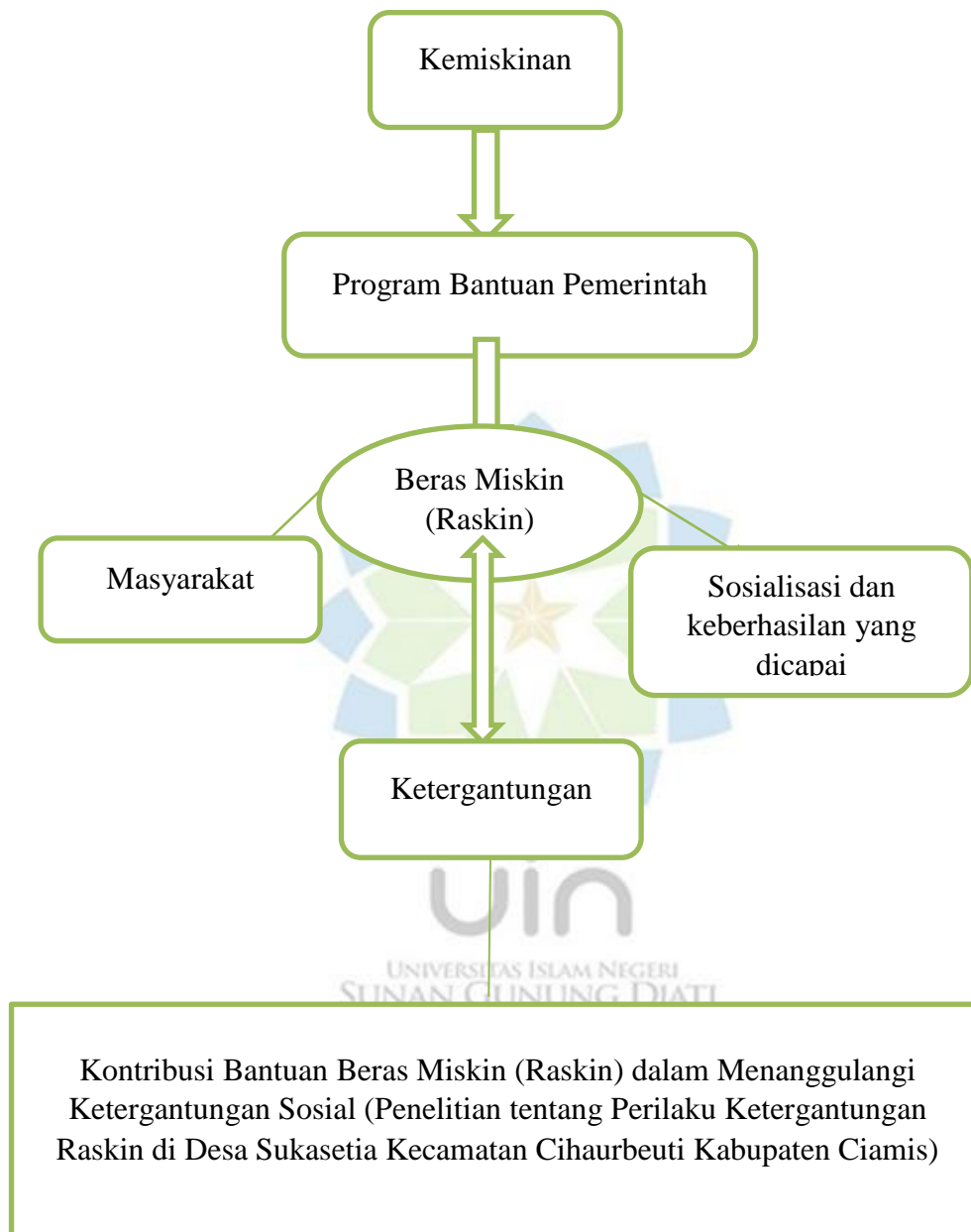
Gambar 1.1 Kerangka Pemikiran
