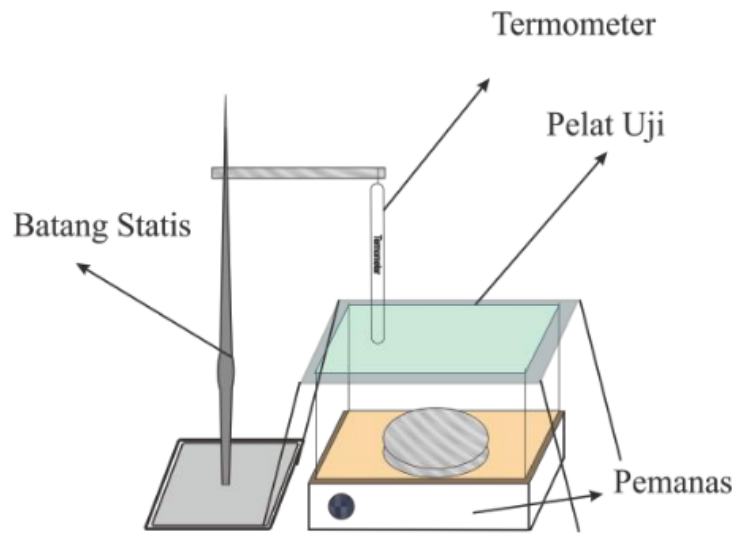
Gambar 1. Set Praktikum Radiasi Kalor
