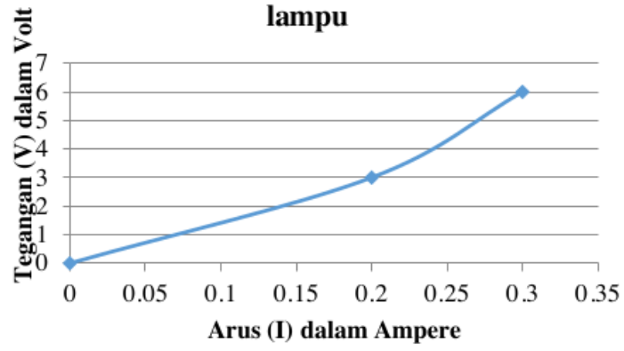
Grafik V terhadap I pada percobaan resistor 47 ohm
