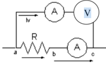
Gambar 1. Pengukuran Arus dan Tegangan
