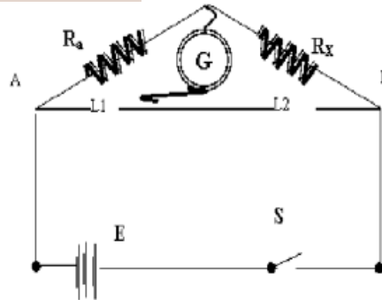
Gambar 4. Rangkaian Jembatan Wheatstone yang Disederhanakan
