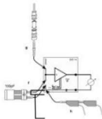
Gambar 2. Susunan Amplifier Untuk Mengukur Batas Tegangan
