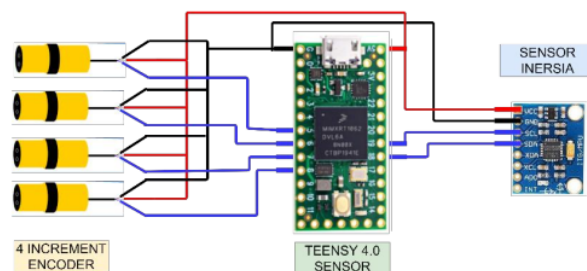
Gambar 2. Rangkaian elektrik eksperimen
