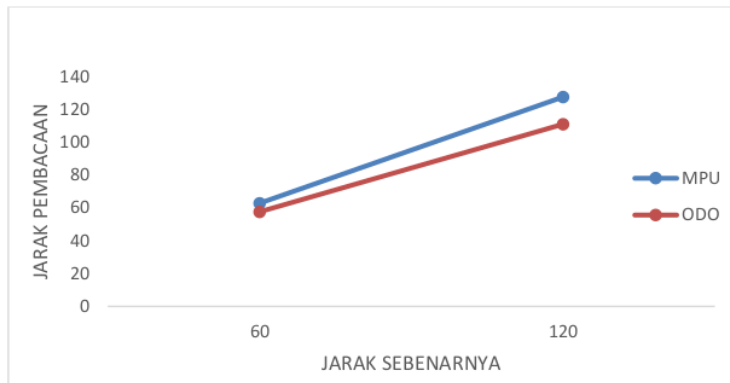
Gambar 6. Perbandingan pembacaan jarak perpindahan antara metode integral euler dengan metode perputaran roda pada kondisi kekiri
