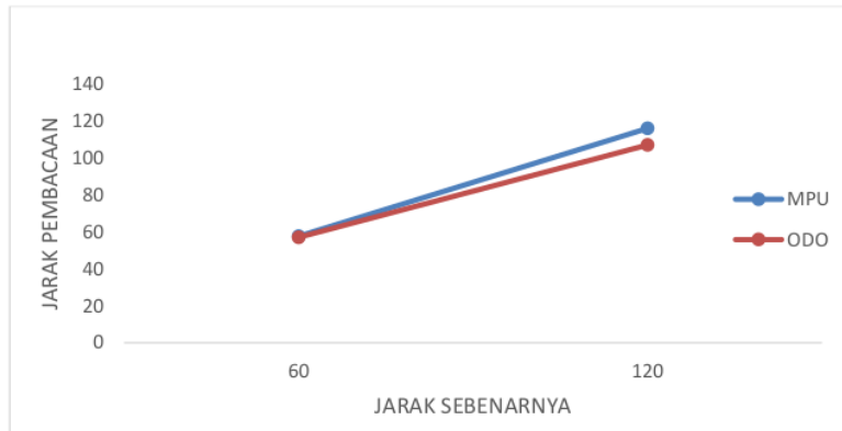
Gambar 5. Perbandingan pembacaan jarak perpindahan antara metode integral euler dengan metode perputaran roda pada kondisi mundur
