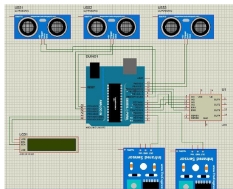
Gambar 5. Konfigurasi sistem secara keseluruhan
