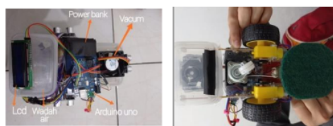
Gambar 8. Tampak robot dari (a) atas; (b) bawah.
