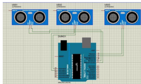
Gambar 4. Konfigurasi sensor ultrasonik
