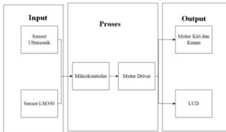
Gambar 1. Blok diagram sistem secara keseluruhan.
