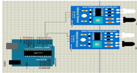
Gambar 3. Konfigurasi sensor LM393
