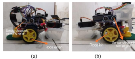
Gambar 7. Tampak robot dari samping (a) kanan; (b) kiri.
