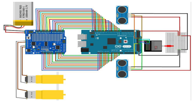
Fig. 2. Schematic robot.
