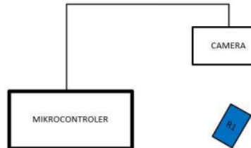
Fig. 4. Dataset RTURNRIGHT
