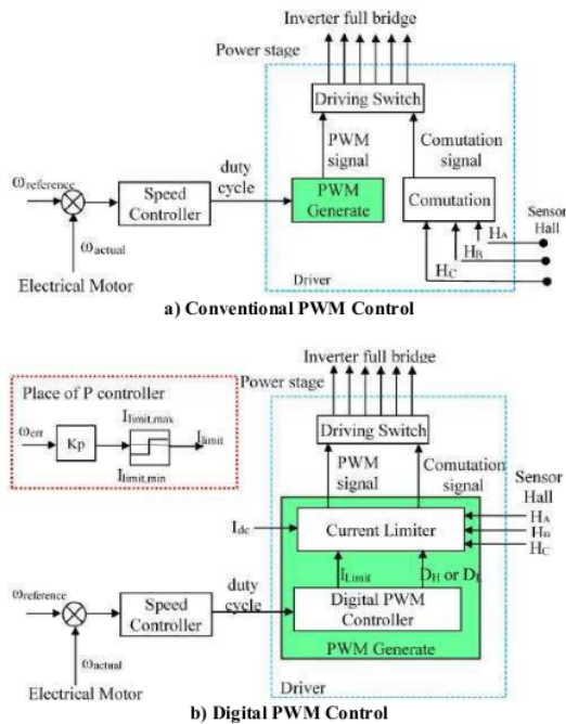
Fig. 6. PWM technique.
