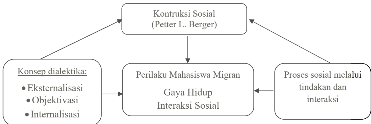
Gambar 1.1 Kerangka Pemikiran
