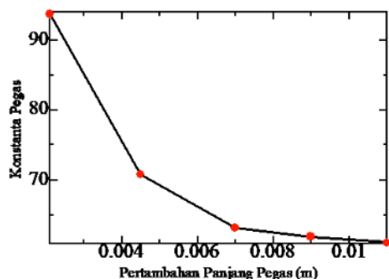
Grafik 5. Percobaan 5 Hubungan Konstanta Pegas dan Panjang Pegas di Bulan
